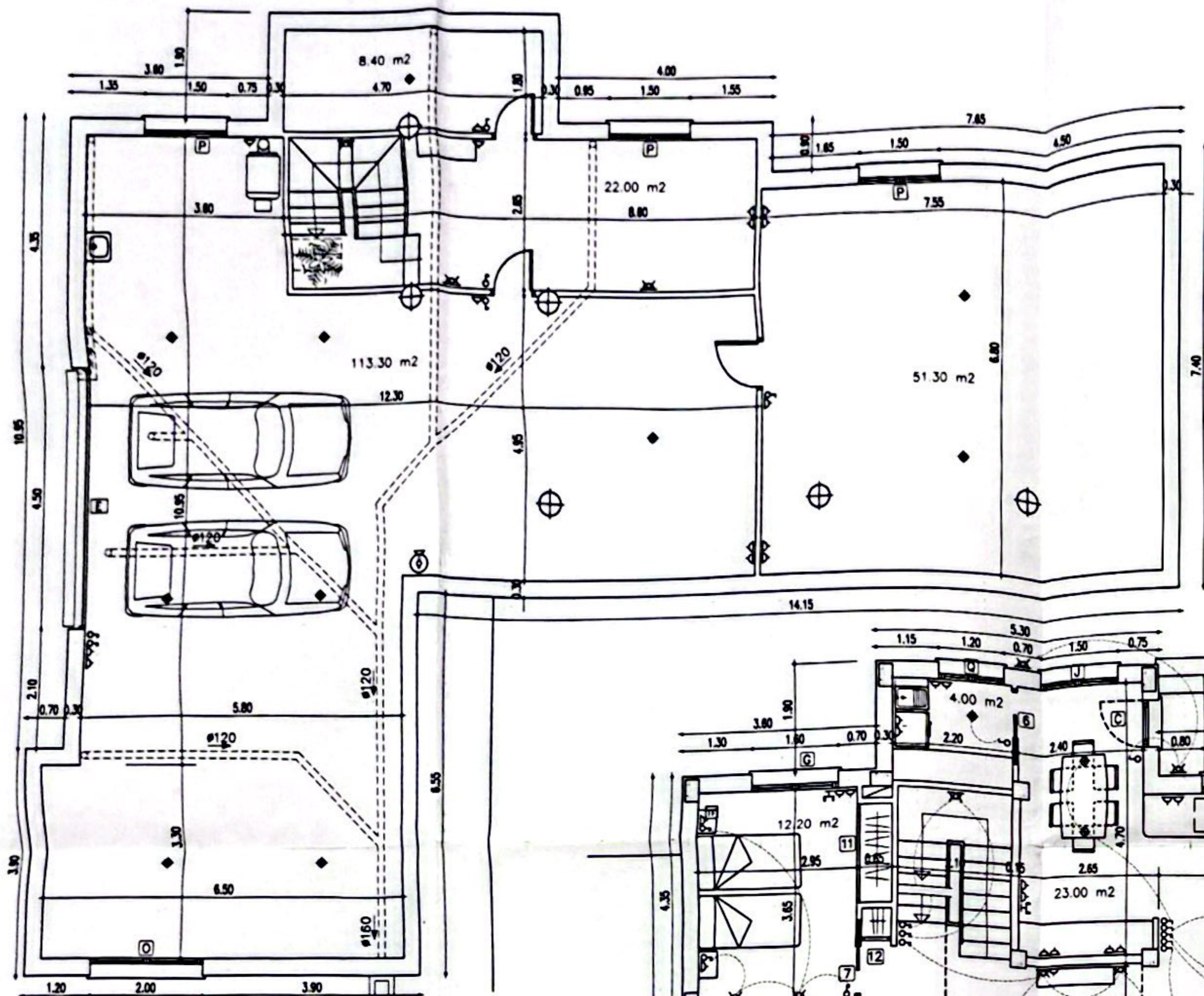
Planta soterrani 1:50 SUPERFICIE CONSTRUÏDA 217.00 M2
